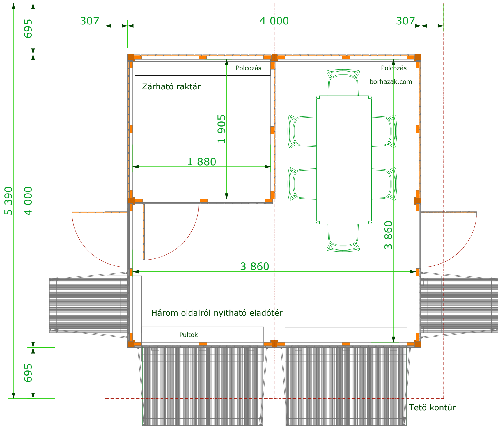
4x4 méteres borház alaprajza II. var.
