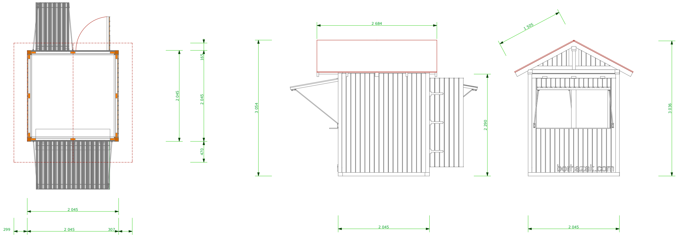
2x2 méteres faház rajzai
