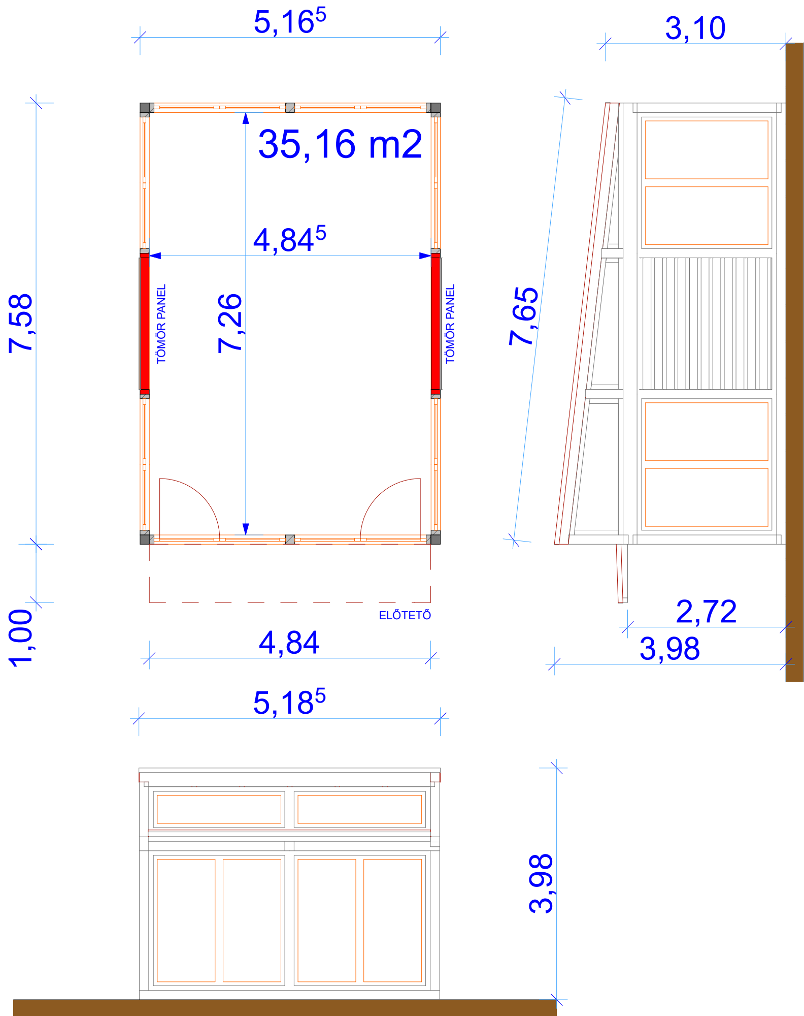
PEZOWOOD Melegedő alaprajza, nézeti rajzai
